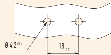
Fixing grid Befestigungsrastrer
